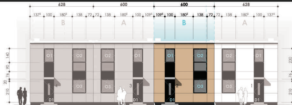
ELEWACJA FRONTOWA
